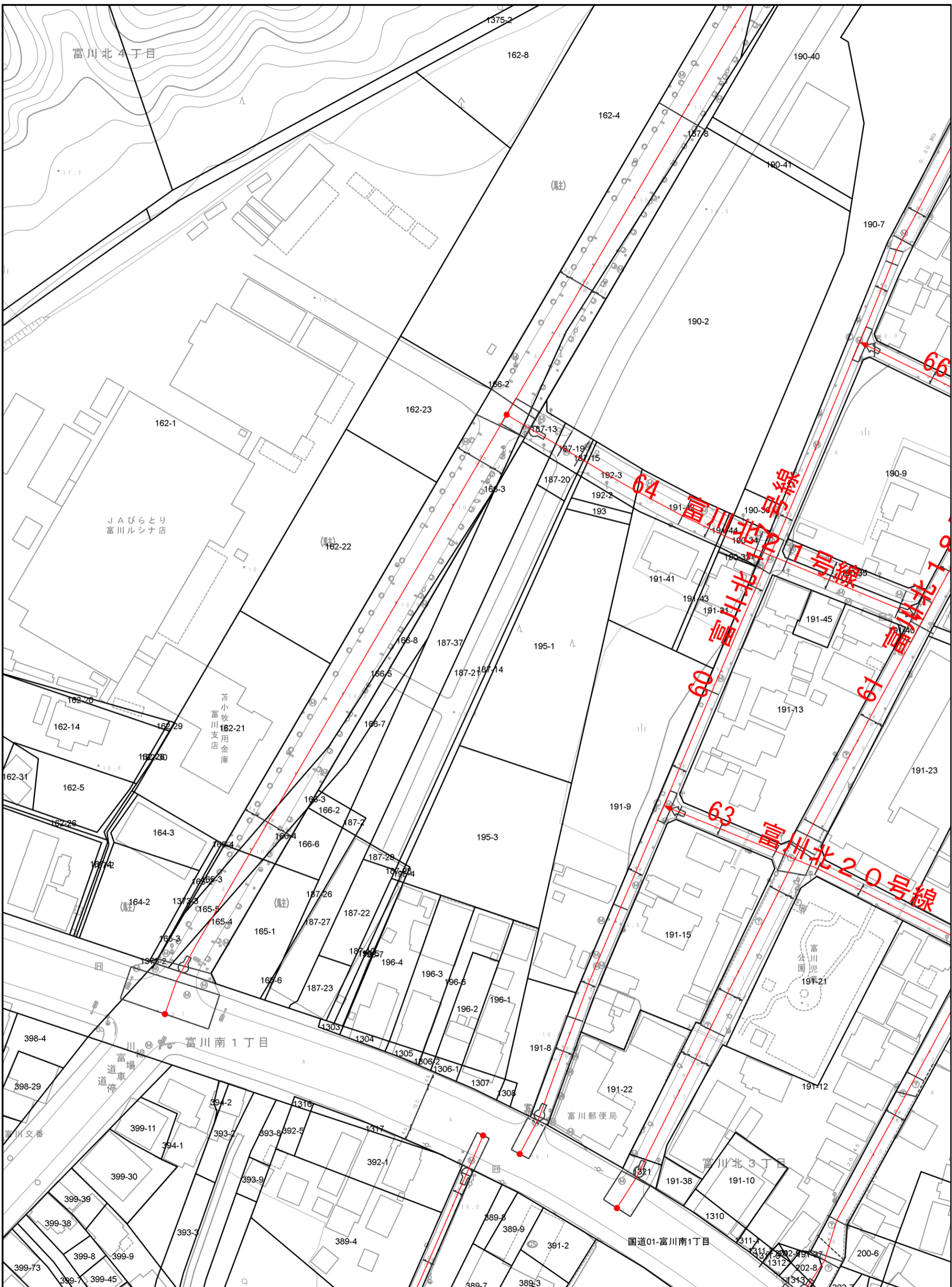
道路台帳図
